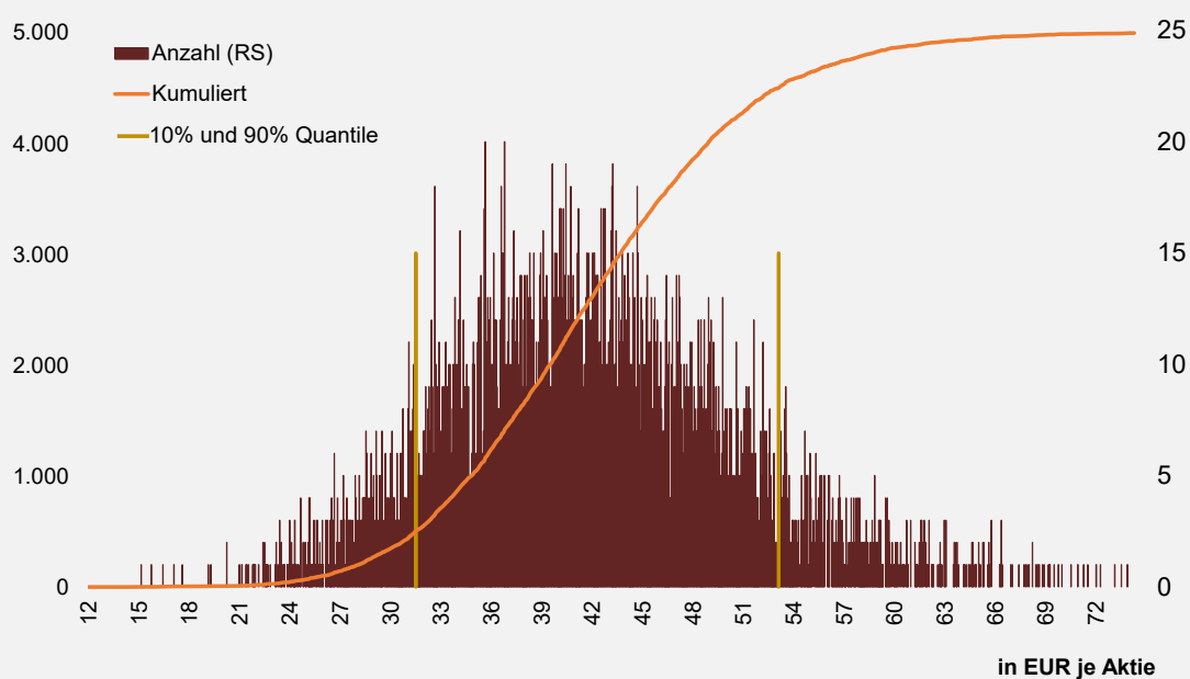
ABBILDUNG 1: MONTE-CARLO-SIMULATION (5.000 SIMULATIONEN)
